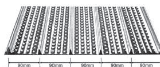
Hy-Rib (2' x 8')
